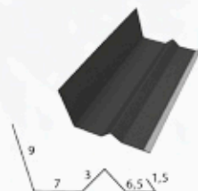
WIATROWNICA PROFILOWANA
