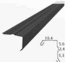
WIATROWNICA PROFILOWANA
