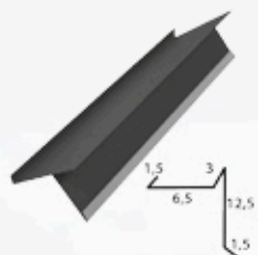
KORYTO PRZYŚCIENNE
